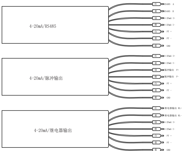
能量表7芯通讯线接线图
