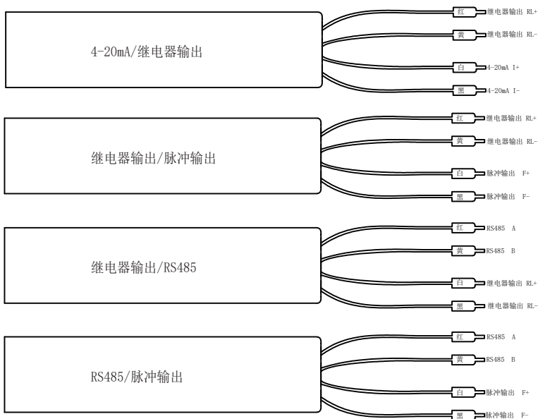
能量表7芯通讯线接线图
